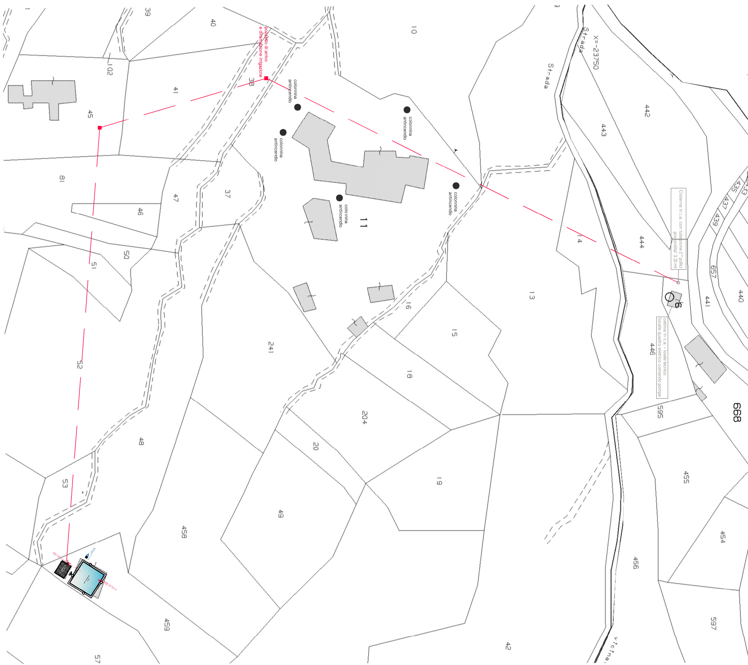
SCHEMA PERCORSO TUBAZIONE
