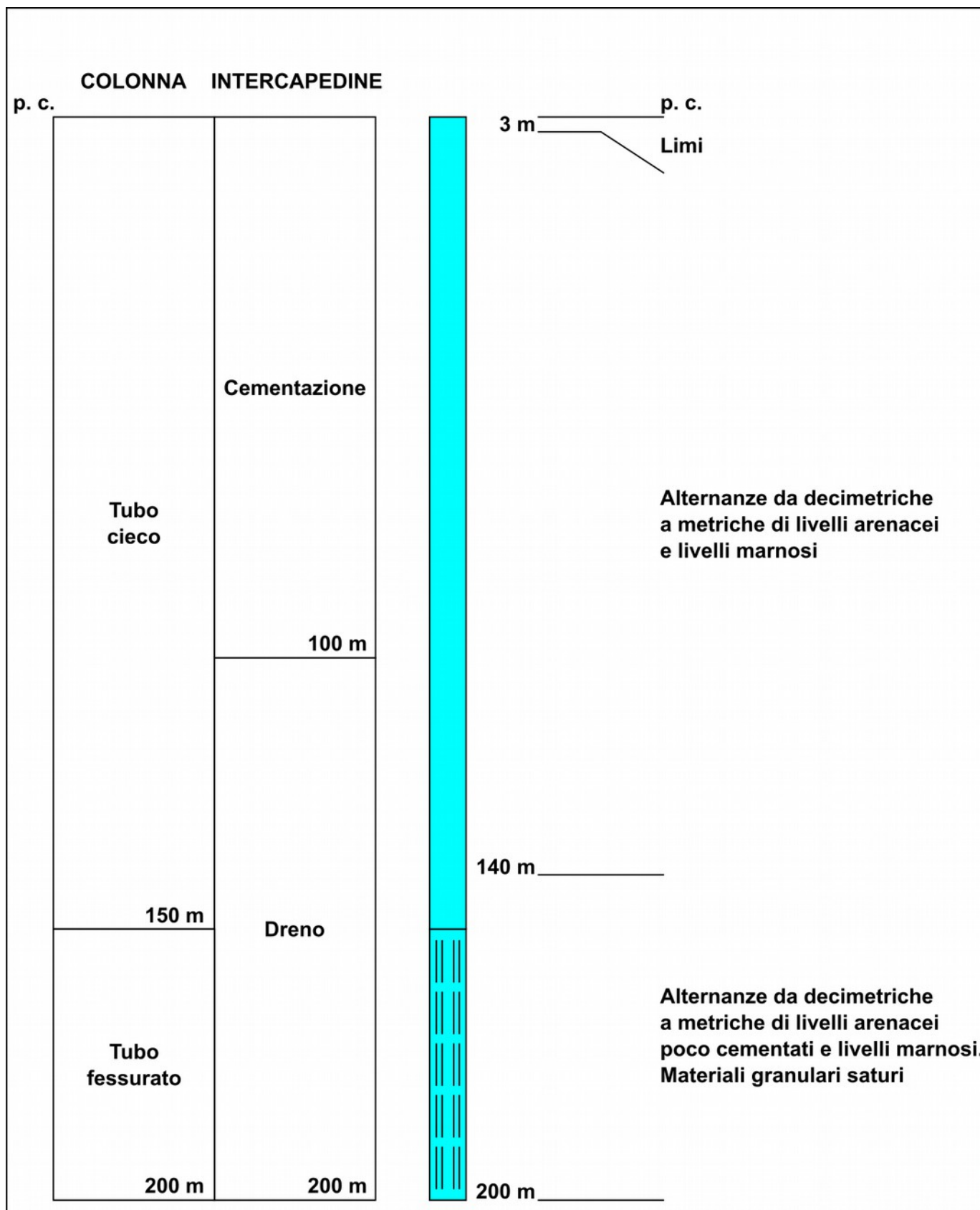
Figura 1 – Stratigrafia e caratteristiche costruttive del piezometro realizzato (scala verticale = 1:1000)
